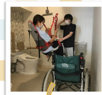
あいじょう 愛移乗くん 2017年より導入
